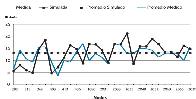
Figura 10. Curva comparativa de presiones. Sector Casco Central.
