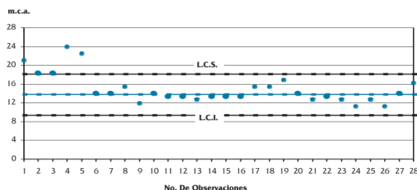
Figura 4. Registros de Presión. La Consolidada. Aguas Arriba.
