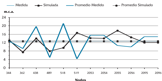
Figura 11. Curva comparativa de presiones. Sector Este.
