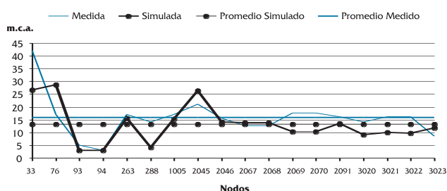
Figura 8. Curva comparativa de presiones. Sector Norte.
