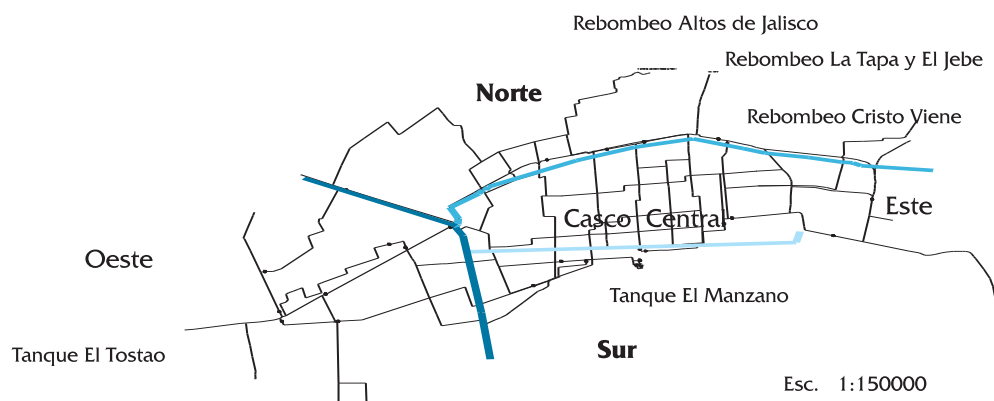
Figura 1. Esquema del Macromodelo la Red de Esc. 1:150.000
