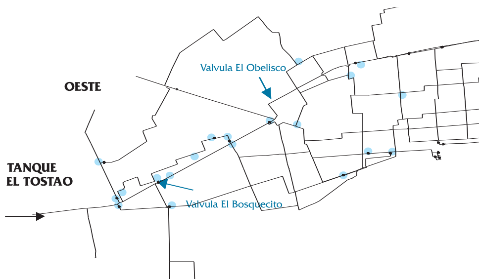
Figura 2. Ubicación de las válvulas “El Obelisco” y “Bosquesito”
