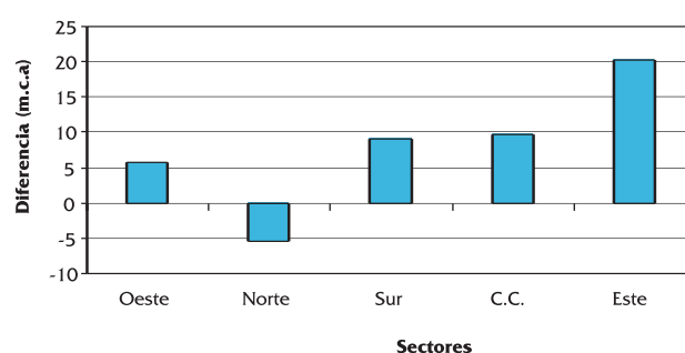
Figura 6. Gráfico de la diferencia del Promedio de Presiones
