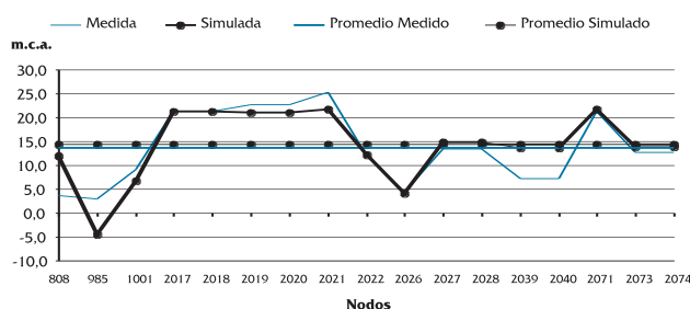
Figura 7. Curva comparativa de presiones. Sector Oeste.
