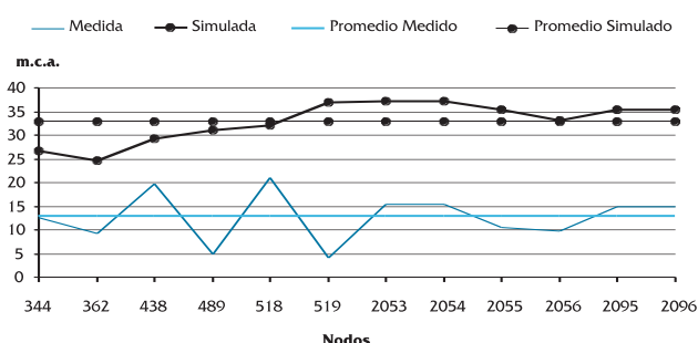
Figura 5. Gráfico de comparación de Presiones. Sector Este.
