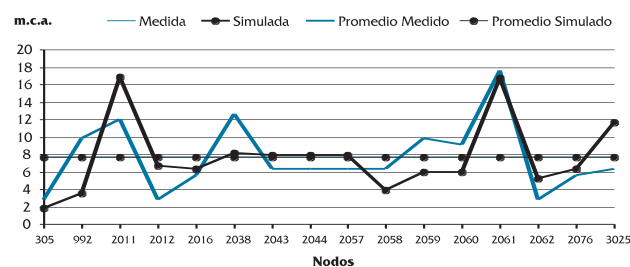
Figura 9. Curva comparativa de presiones. Sector Sur.
