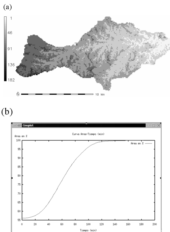
Figura 11. Tiempos de viaje del flujo. MDE 50 m. V_{\text{media}}=30\text{m/min} [1,300]m/min: (a) Mapa reclasificado para \Delta t=30 min y (b) Curva Área-Tiempo obtenida desde el mapa original.
