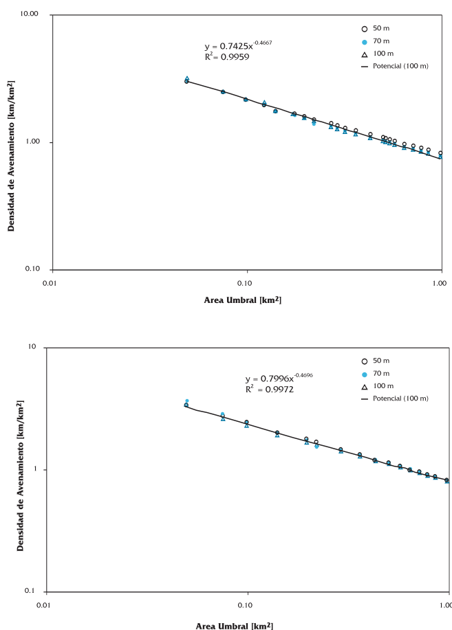
Figura 1. Ajuste de Ley Potencial. Relación D_d - A_{\text{umbral}} : (a) Cca. Corneros y (b) Cca. Rbla. Salada.
