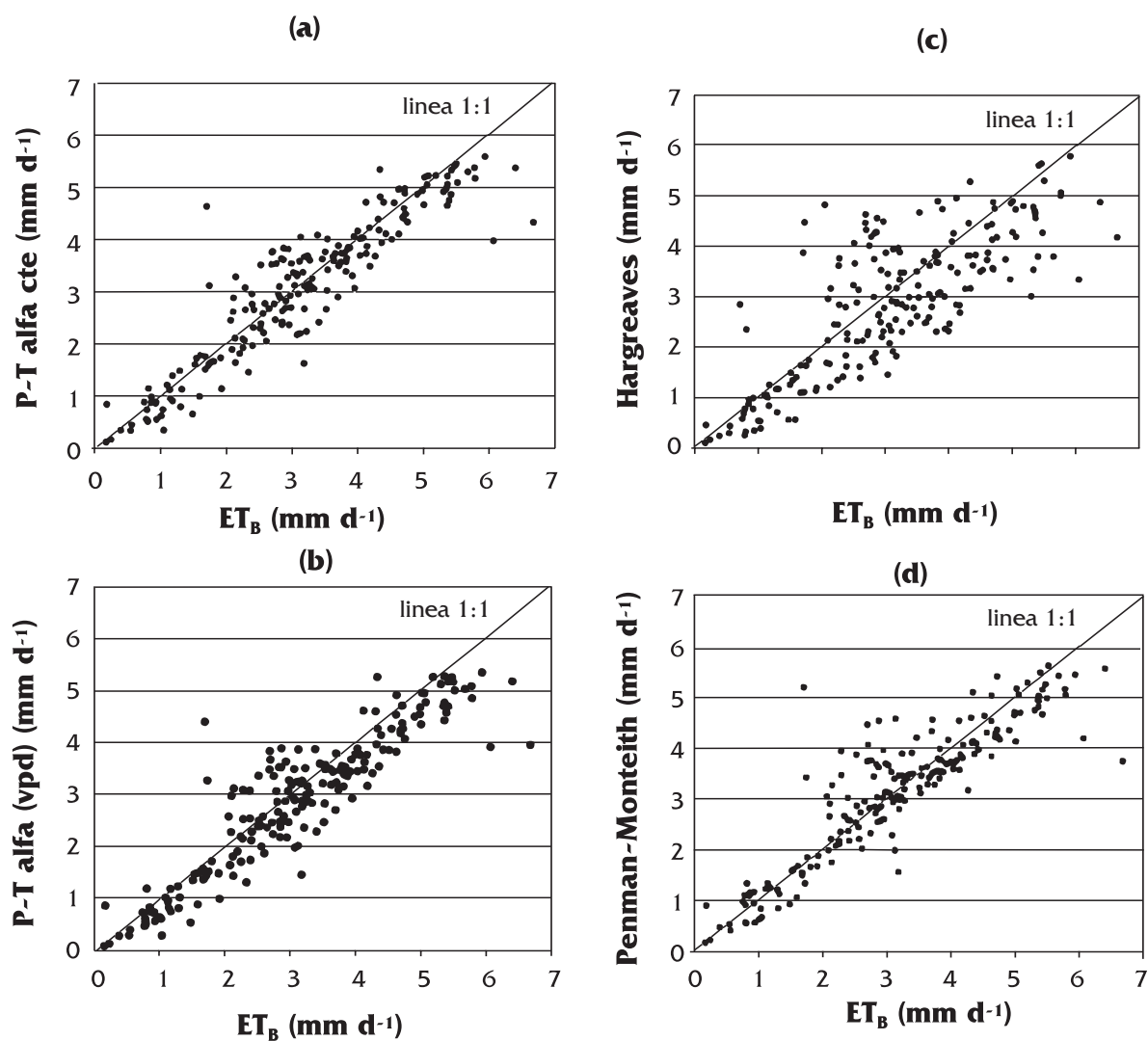
Figura 3. Estimación de ETo ( mm\ d^{-1} ) mediante la ecuación de Priestley-Taylor con \alpha constante (a), con \alpha dependiente del DPV (b), mediante la ecuación de Hargreaves (c), y mediante la ecuación de Penman-Monteith (d) con respecto a la evapotranspiración medida ( ETB ) para todo el conjunto de datos diarios.
