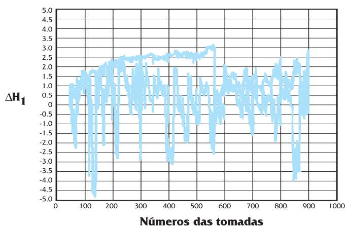
Figura 2. Curvas envolventes dos défices de pressão relativa simulados para as tomadas do sistema de rega de Sinistra Ofanto, Capitanatta, Foggia, Itália, para um caudal total Q_r = 1200 \text{ l s}^{-1} . As simulações foram realizadas com geração aleatória da procura e recorrendo a 1000 configurações de 120 tomadas abertas em simultâneo. Fonte: Lamaddalena e Pereira (1998).
