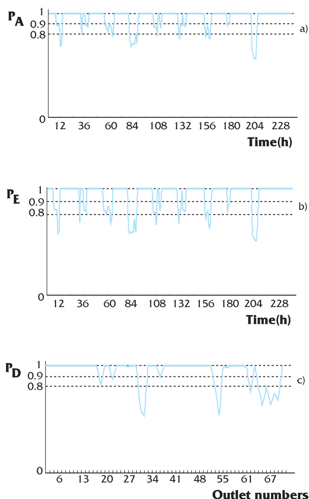
Figura 1. Fiabilidade (a), equidade (b) e regularidade (c) no fornecimento de caudais nas tomadas da rede de distribuição em baixa pressão do sector 11 do sistema de rega do Vale do Sorraia durante o decêndio de ponta (as linhas horizontais referem-se aos limites de desempenhos considerados muito bom e bom). Fonte: Douieb et al. (1998).
