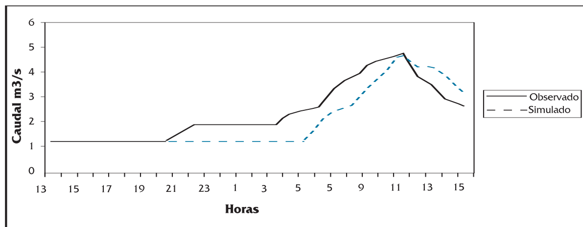
Figura 5. Comparación del hidrograma observado y simulado 13/14-VI-1992
