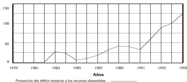
Figura 4: Proporción del déficit (sobreexplotación global de acuíferos) respecto a los recursos renovables disponibles. En 1994 el volumen de sobreexplotación es equivalente a la totalidad de los recursos renovables disponibles. (Valor expresado en tanto por ciento)
