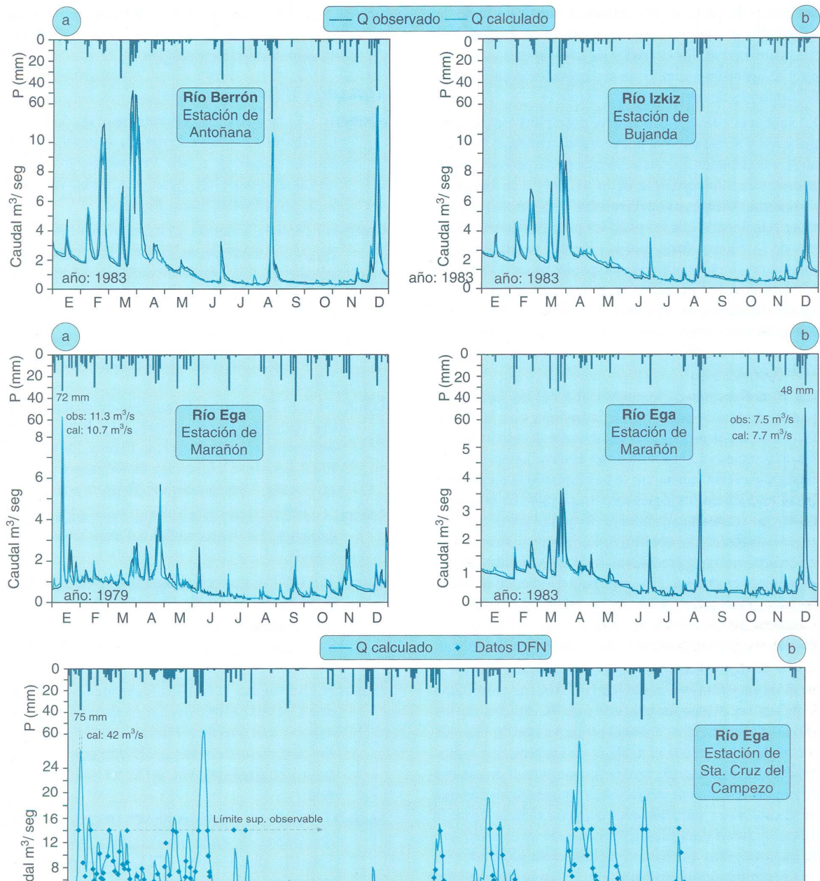
Figura 5. Hidrogramas observados y calculados: a. calibración y b. validación
