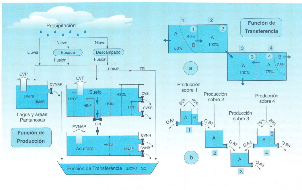
Figura 3. Funciones de producción y de transferencia del modelo Cequeau
