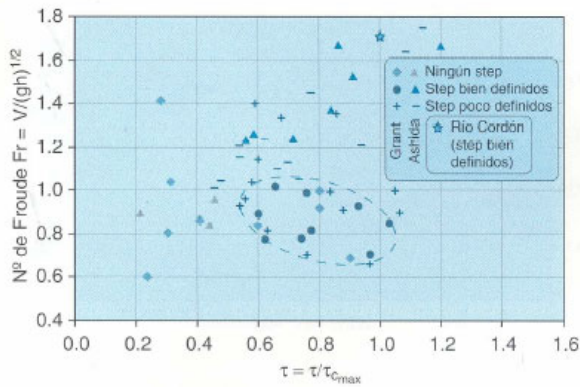
Figura 4. Dominio de deformación de los escalones (Grant, 1994) ne también los datos de laboratorio de Ashida y otros (1984), la abscisa representa el parámetro adimensional \tau^* (dado por la relación entre el esfuerzo de tracción medio ( \tau ) y el esfuerzo de tracción máximo ( \tau_{Cmax} ) ne-
