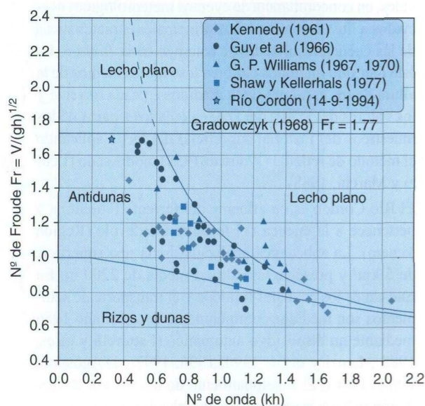
Figura 3. Configuraciones de fondo según Allen (1982)
