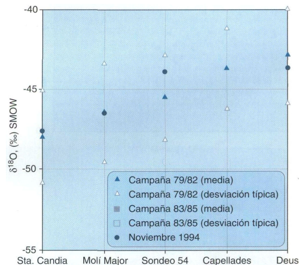
Figura 4. Valores isotópicos ( \delta^{18}\text{O} y \delta\text{D} ) correspondientes a las campañas de muestreo 1979-82, 1983-85 y noviembre de 1994. Para las campañas 1979-82 y 1983-85 se ha representado tanto el valor medio como la desviación típica. Puntos de muestreo: Lago de Capellades, Sondeo S4 (Capellades), Les Deus, Mina del Molí Major y Santa Candia. Durante noviembre de 1994 no se muestreó el Lago de Capellades
