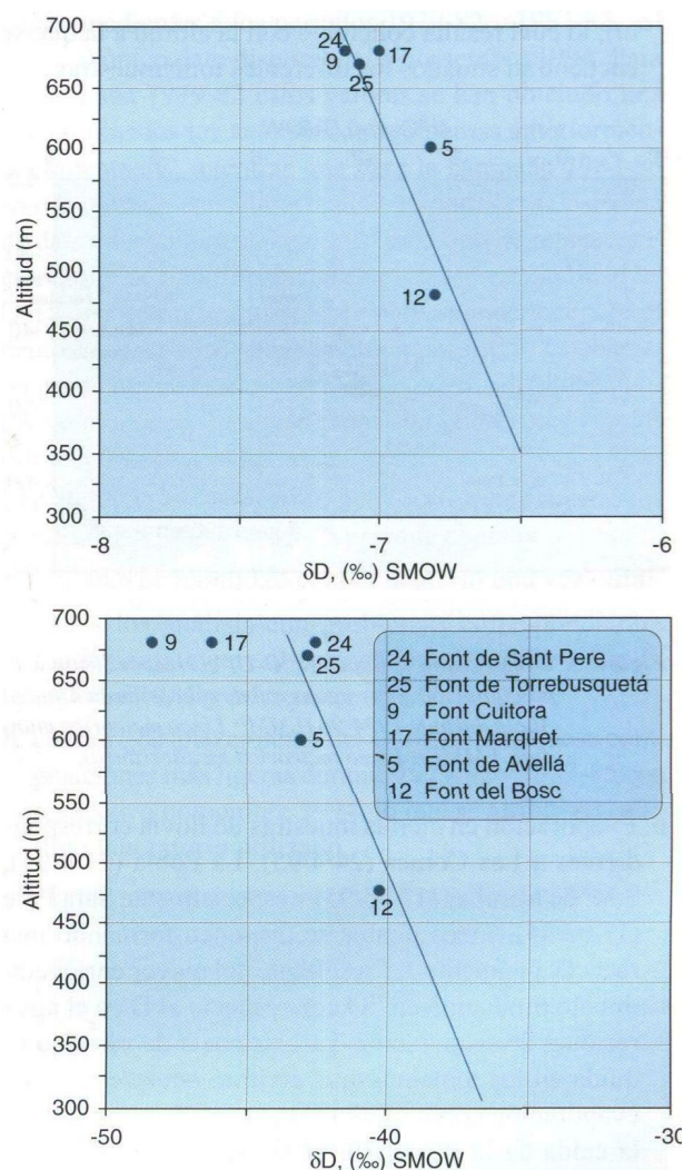
Figura 7. Rectas altitudinales locales obtenidas para el O^{18} -D a partir de manantiales que representan razonablemente bien la cota de recarga del sistema. Datos correspondientes al periodo 1994-96
