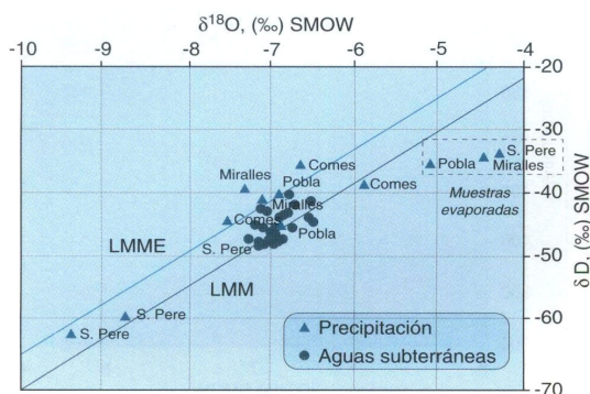
Figura 5. Composición isotópica ( ^{18}\text{O} -D) correspondiente a la precipitación y las aguas subterráneas de la Unidad Anoia durante 1994-96 (LMM= Línea meteórica mundial; LMME= Línea meteórica mediterránea).
