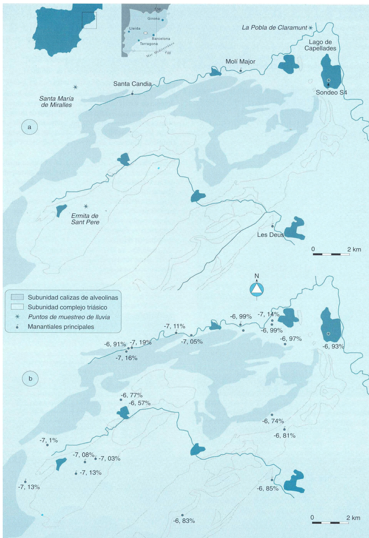
Figuras 1a y 1b. (1a.) Mapa de situación de la Unidad Anoia (Cordillera Prelitoral Catalana): puntos de muestreo de lluvia y principales manantiales considerados. (1b.) Mapa de distribución de \delta^{18}\text{O} en el agua subterráneas correspondiente al muestreo realizado durante el periodo 1994-96. Valores en ‰ SMOW
