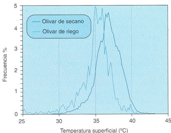
Figura 10. Histograma temperatura superficial para el olivar
