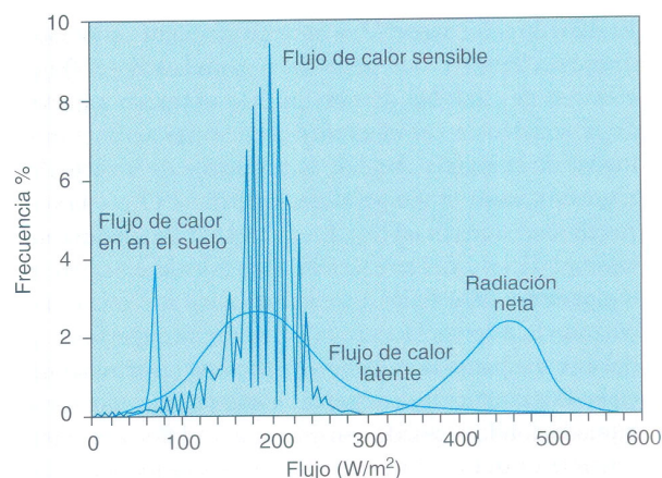
Figura 6. Flujos de calor
