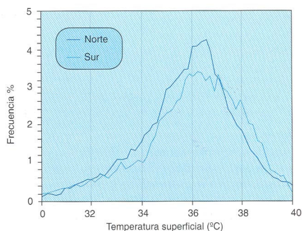
Figura 8. Histogramas de temperatura superficial para las orientaciones norte y sur
