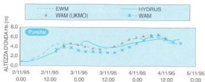
Figura 7: Serie temporali della altezza significativa nel punto Parsifal, ottenute con differenti combinazioni di modelli meteorologici e di moto ondoso.
