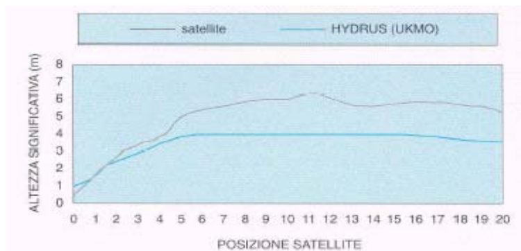
Figura 9: Confronto tra l'altezza significativa calcolata con il modello HYDRUS e le misure del satellite Topex, lungo la traiettoria riportata in figura 3 (posizioni ogni 20 km circa).
