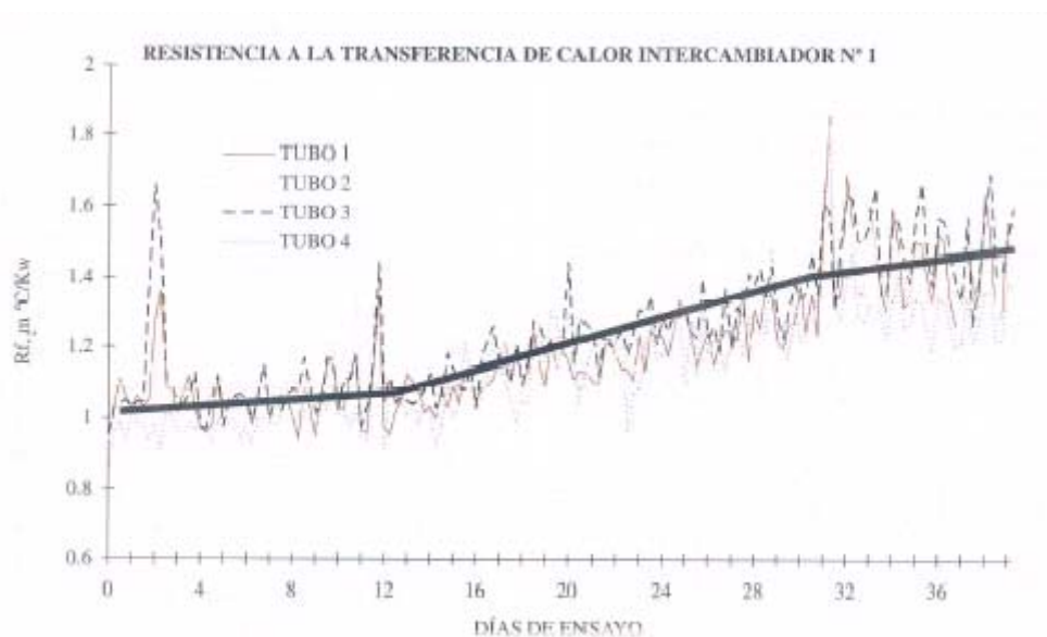
Figura 8. Resistencia a la transferencia de calor para los tubos del intercambiador N° 1, para los 39 días de crecimiento de biopelícula.
