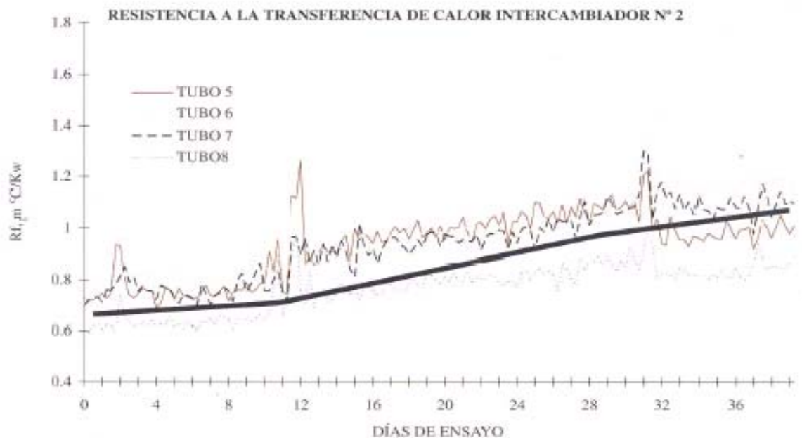
Figura 9. Resistencia a la transferencia de calor para los tubos del intercambiador N° 2, para los 39 días de ensayo.
