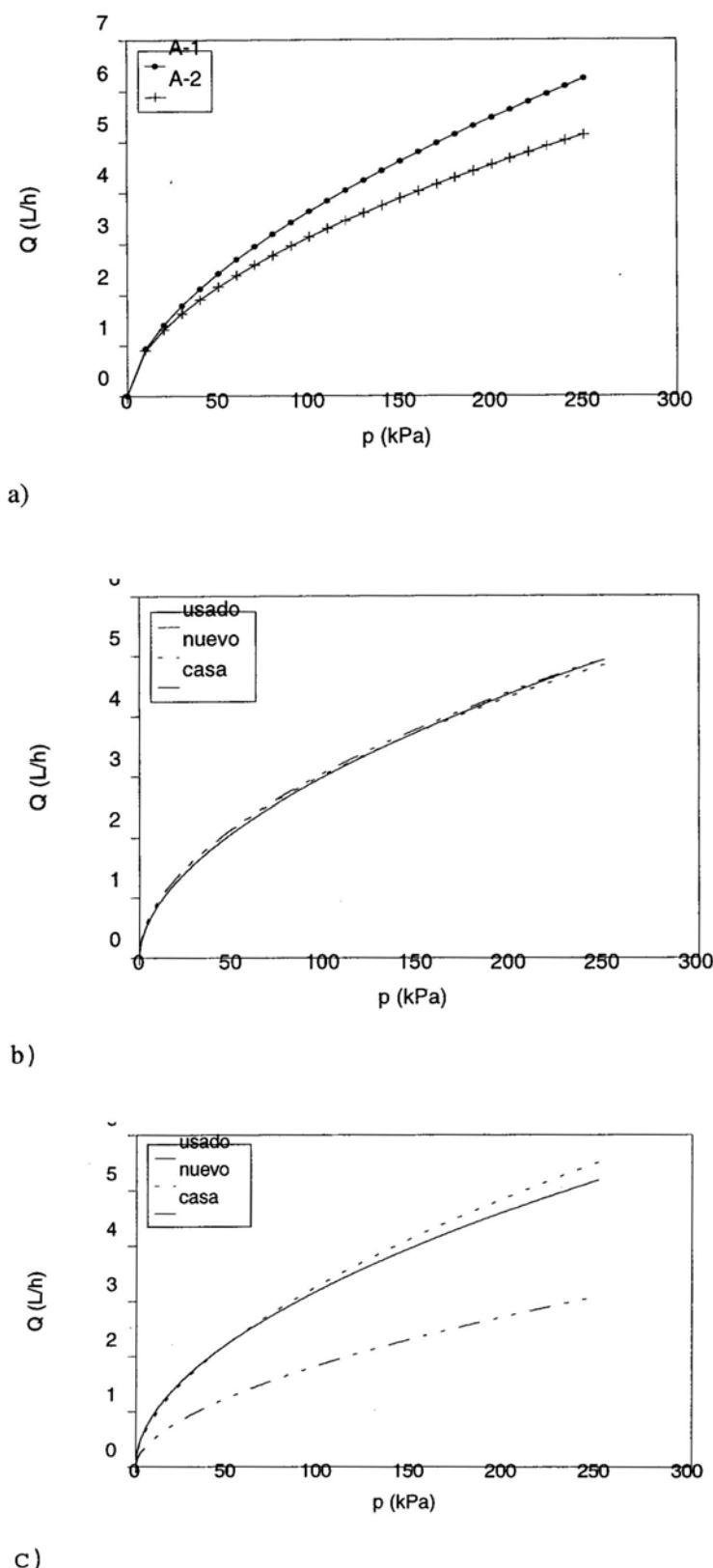
Figura 4. Curvas de gasto de goteros: a) nuevos; b) usados con marca de calidad; c) usados de baja calidad
