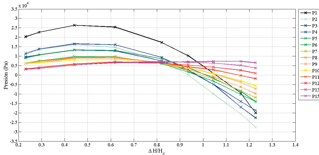
Figura 4 | Evolución de las presiones sobre el paramento en el aliviadero original según el modelo físico.
