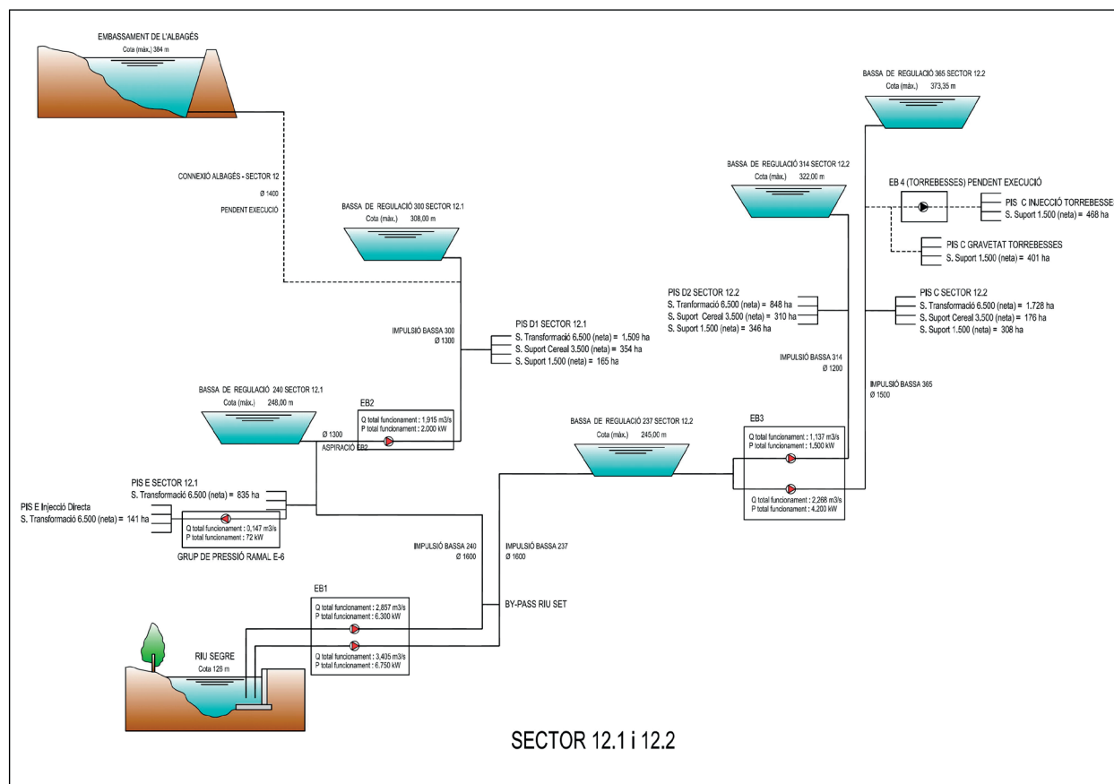
Figura 3 | Esquema sector 12.
