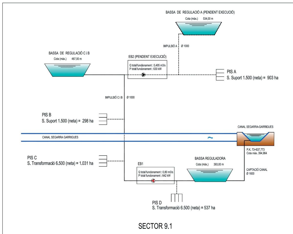
Figura 4 | Esquema sector 9.1.
