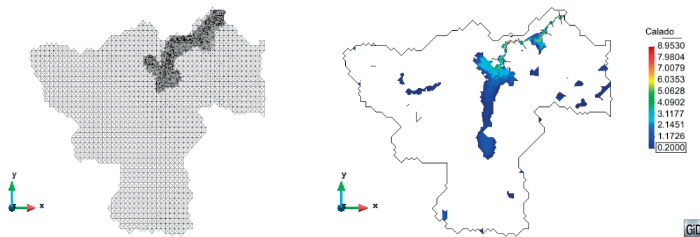
Figura 4 | Malla de cálculo (izquierda) y mapa de inundabilidad (derecha) para la cuenca de cabecera del río Fluvà realizado mediante modelización integrada hidráulico-hidrológica.
