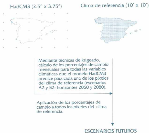
Figura 1. Metodología para la interpolación de los valores del modelo HadCM3 al clima de referencia
