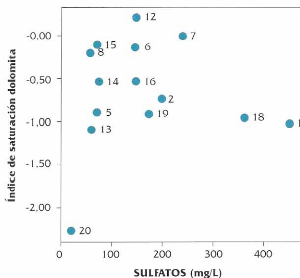
Figura 7. Relación entre el índice de saturación de la dolomita y el contenido en sulfatos.
