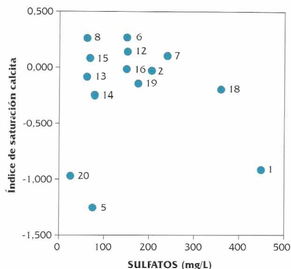
Figura 6. Relación entre el índice de saturación de la calcita y el contenido en sulfatos.
