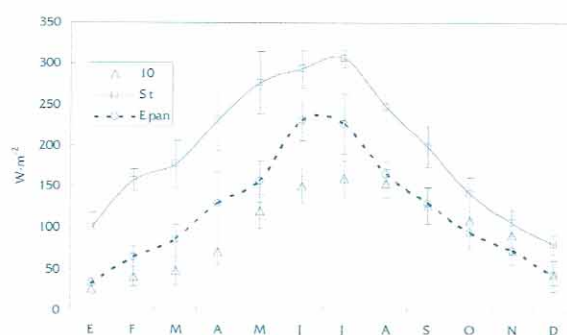
Figura 6. Evolución de la radiación solar S_t , E_{pan} y E_{res} en un embalse de 10000 m 2 y 10 m de profundidad
