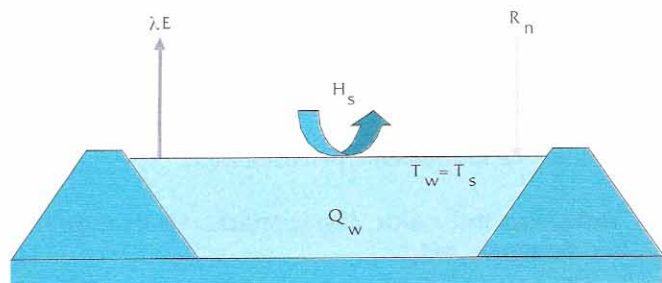
Figura 1. Esquema de los flujos energéticos que intervienen en el balance de un embalse de riego con comportamiento isoterma
