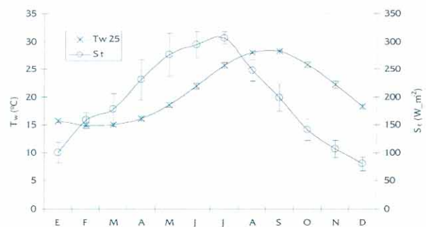
Figura 4. Evolución de la radiación solar S_r , y de la temperatura del agua T_w , para un embalse de 10000 m 2 y 25 m de profundidad
