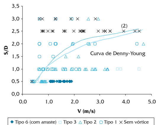
Figura 8. Gráfico de S/D em função da velocidade na tomada para os diferentes tipos de vórtices.
