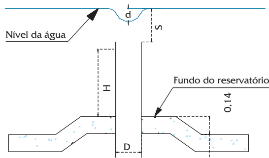
Figura 5. Representação esquemática das variáveis na tomada d'água vertical.
