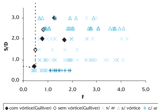
Figura 7. Gráfico comparativo de S/D em função do número de Froude, para tomadas verticais.
