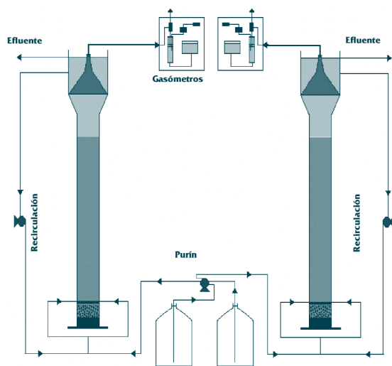
Figura 1: Montaje experimental de los reactores anaerobios de lecho fluidizado.
