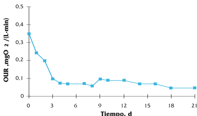
Figura 4. Evolución de la tasa de respiración (OUR) en el ensayo sin aporte de alimentación.
