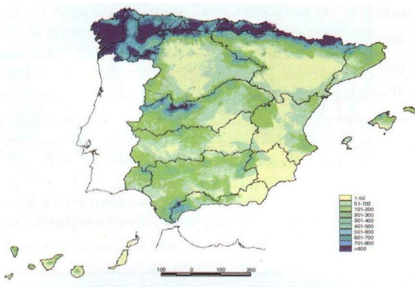
Figura 31. Mapa de escorrentía total media anual en mm (periodo 1940-1995)
