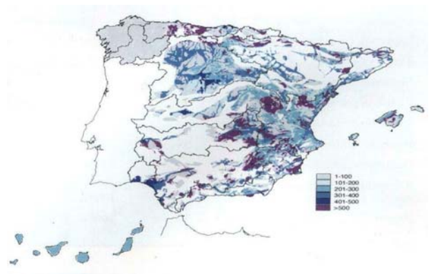
Figura 18. Mapa de capacidad de infiltración máxima (mm)
