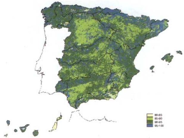
Figura 14. Coeficiente reductor (x100) de la evapotranspiración potencial según el uso del suelo
