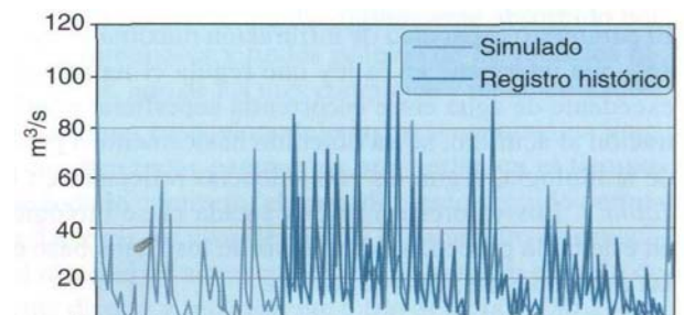
Figura 28. Series mensuales simuladas e históricas del río Tajo en Entrepeñas (periodo 1940 a 1995)
