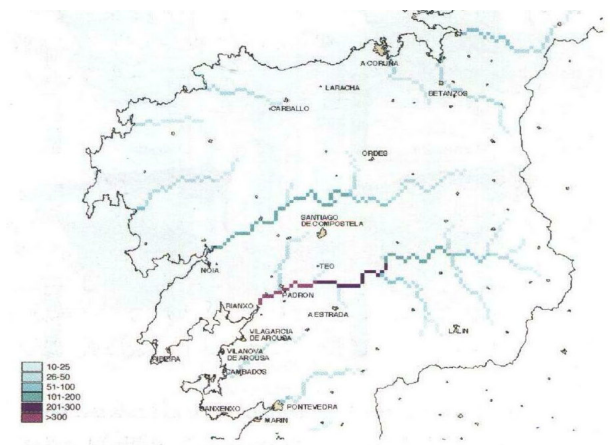
Figura 35. Detalle del mapa de aportaciones en la red fluvial (hm³/mes) en la zona de Galicia (febrero 1970)
