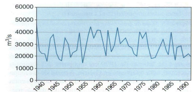
Figura 39. Recarga por infiltración de lluvia (hm³/año) en la Península (periodo 1940/41 a 1995/96)
