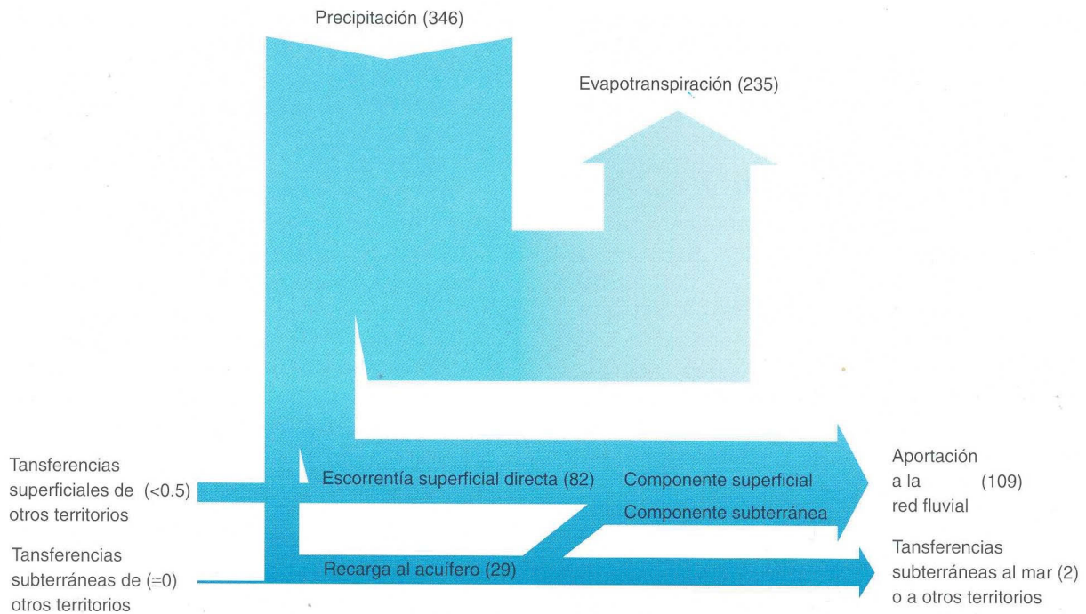
Figura 40. Esquema con los principales flujos de agua (km 3 /año) en España (periodo 1940-1995)
