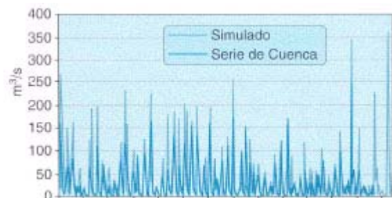
Figura 22. Series mensuales simuladas e históricas del río Alberche (periodo 1940 - 1995)
