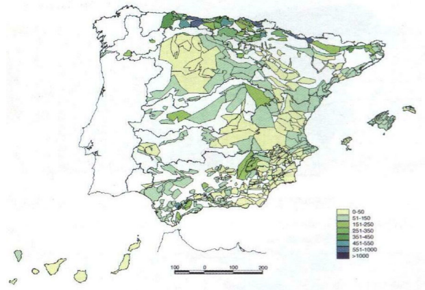
Figura 36. Mapa de recarga natural (infiltración por lluvia directa) en las unidades hidrogeológicas (mm/año)
