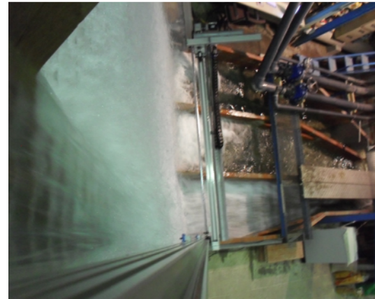
Ilustración 3. Canales de recogida para aforo
